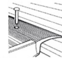
B- Bolzensicherung (Löcher Ø 12 mm)
